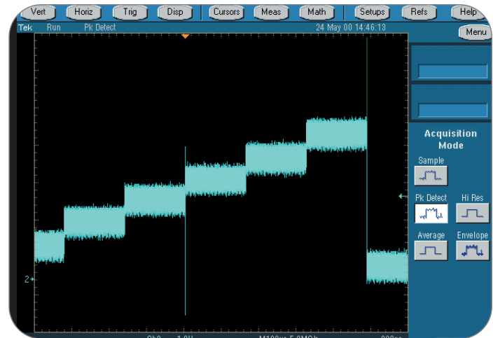
► Abbildung 27. Mit dem Spitzenwerfungsmodus kann das Oszilloskop der TDS7000-Serie nicht repetierende Anomalien mit Breiten bis zu 100 ps erfassen
