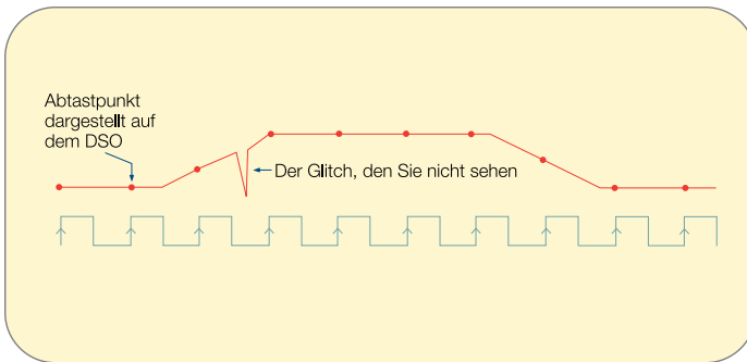
► Abbildung 26. Die Abtastrate ändert sich mit den Zeitbasis-Einstellungen – je langsamer die Zeitbasis-Einstellung, desto langsamer ist die Abtastrate. Einige Digital-Oszilloskope bieten einen Spitzenwerfungsmodus zum Erfassen schneller Transienten bei niedrigen Ablenkgeschwindigkeiten
