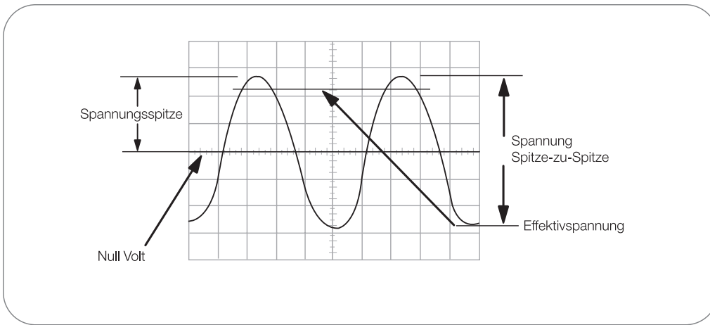
► Abbildung 66. Spannungsspitze ( V_p ) und Spitze-zu-Spitze-Spannung ( V_{p-p} )
