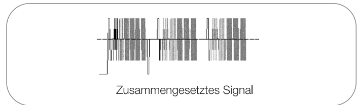
► Abbildung 9. Ein NTSC-Composite-Videosignal ist ein Beispiel eines zusammengesetzten
