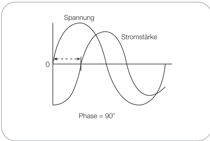
► Abbildung 12. Phasenverschiebung
