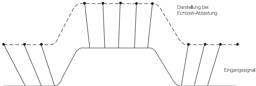
► Abbildung 30. Damit dieser 10-ns-Impuls in Echtzeit erfasst werden kann, muss die Abtastrate hoch genug sein, um die Flanken genau zu definieren
