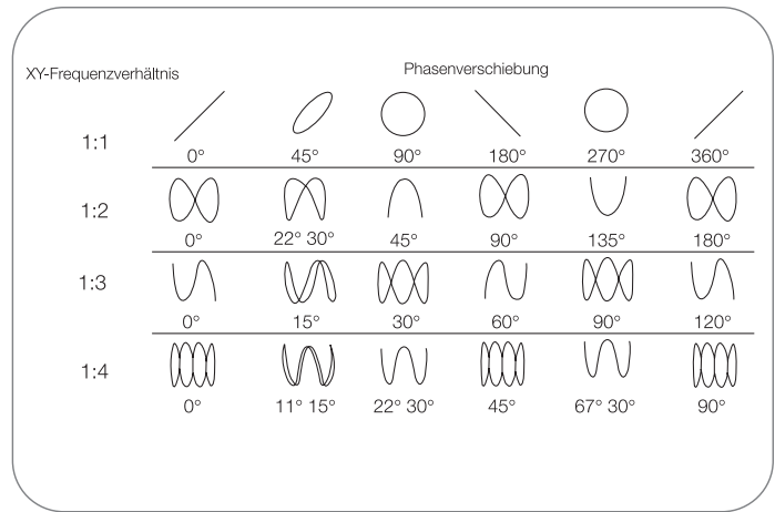
► Abbildung 70. Lissajous-Figuren
