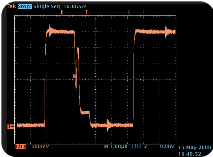
► Abbildung 50. Eine höhere Abtastrate liefert eine bessere Signalaufklärung und stellt sicher, dass Sie intermittierende Ereignisse darstellen können
