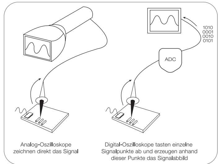
► Abbildung 15. Analog-Oszilloskope zeichnen Signale direkt, während Digital-Oszilloskope Signalepunkte abtasten und daraus Signalabbilder erzeugen
