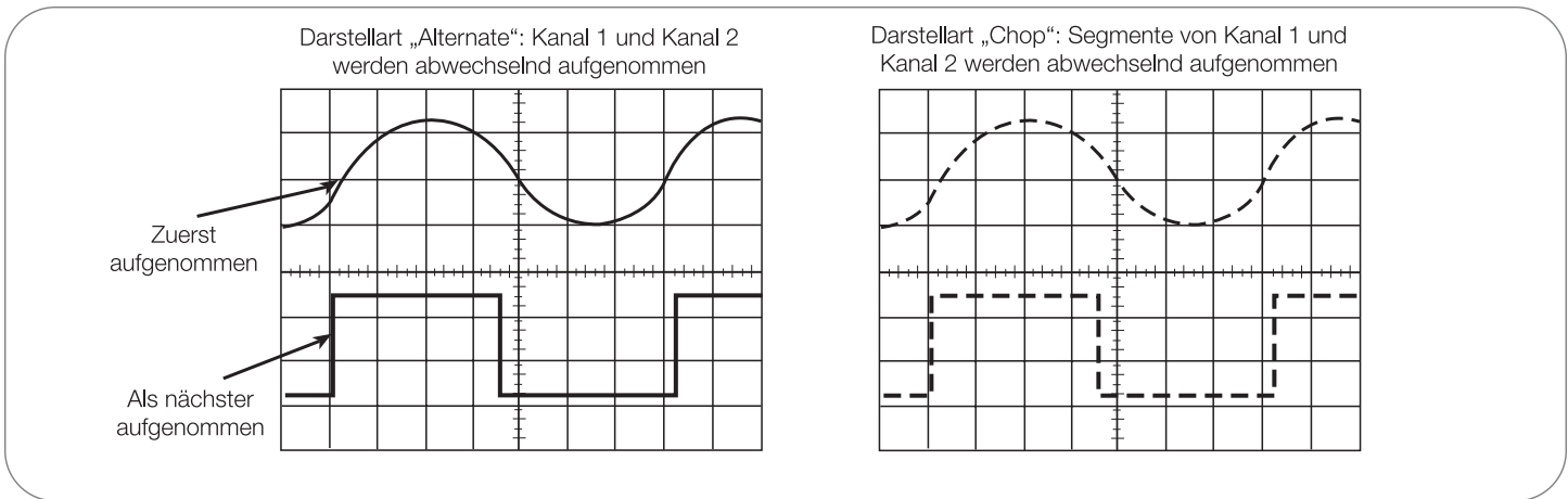
► Abbildung 24. Mehrkanal-Darstellarten
